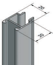
Coulisse 20x20 Type C profil d'éloignement Pose FACE (clips fournis)
