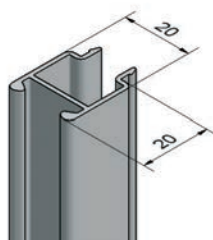
Coulisse 20x20 Type C profil d'éloignement Pose FACE (clips fournis)
