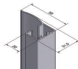
Coulisse 55x31,5x20 Type H Pose en BAIE ou pose FACE intérieure ou extérieure
