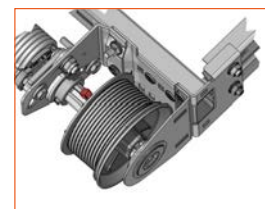
Fixation ligne d'arbre arrière sur rail horizontal, linteau réduit (100/120mm)
